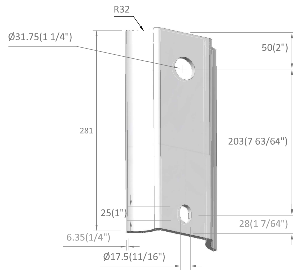
DETALLE B ISOMÉTRICO SOPORTE Escala 1:5
